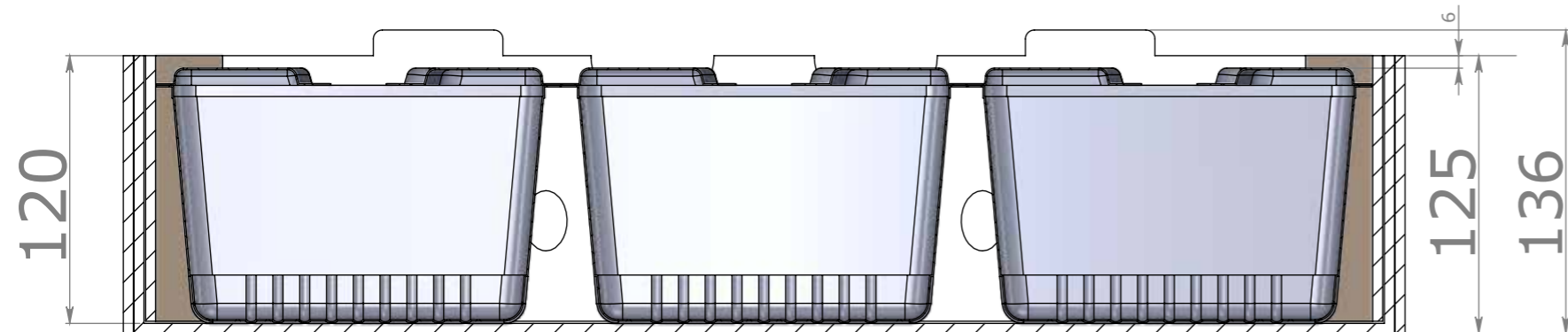
SECTION A-A
